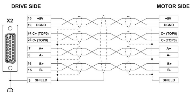
FIG. 27- X2 collegamenti Sin Cos Incrementale / X2 Incremental Sin Cos connections
