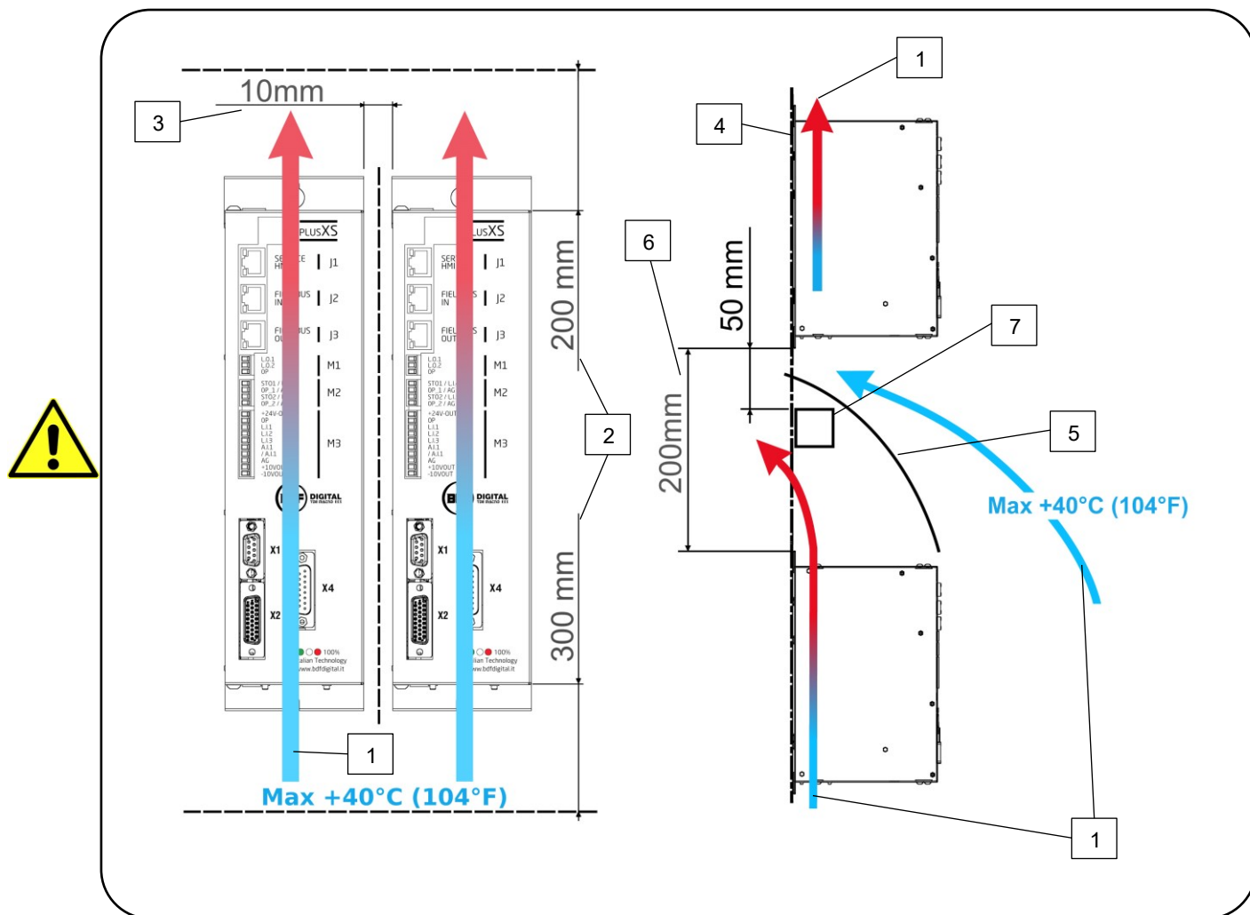
FIG. 13- Installazione / Installation
